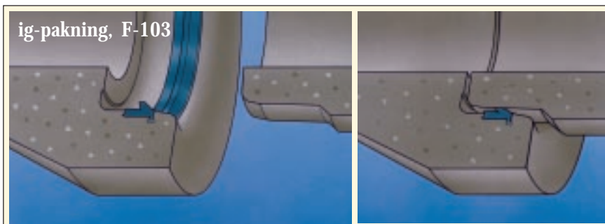
Snit i betonrørssamling med ig-pakning, henholdsvis før og efter samling.
